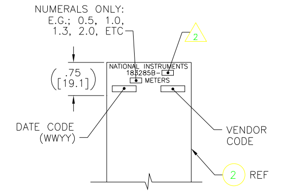
DETAIL B SCALE: NONE
